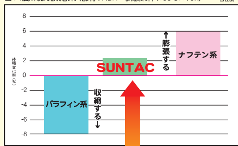
ゴム膨潤試験結果(部材:NBR 試験条件:150°C×70h) 自社調べ
